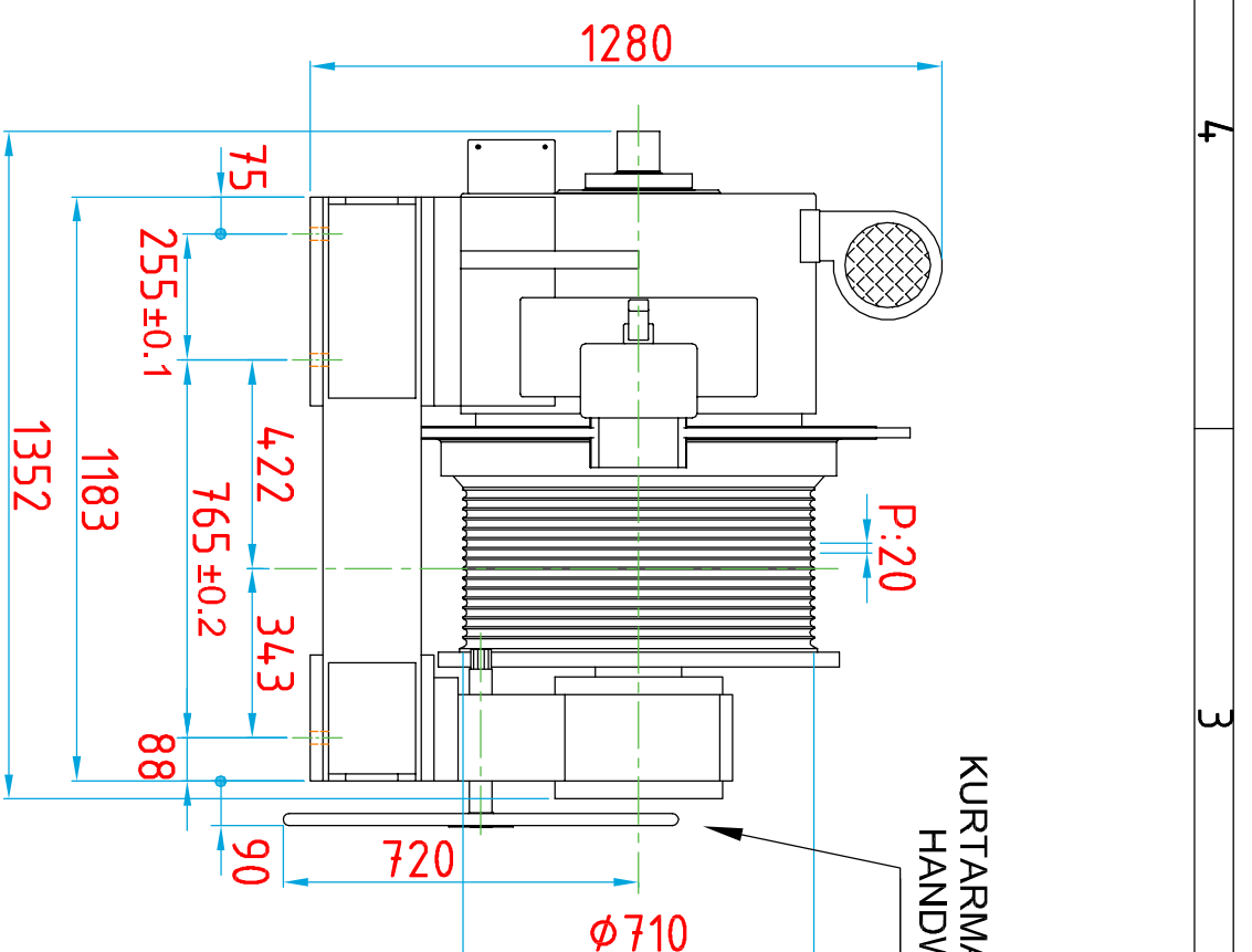
YAN GÖRÜNÜŞ/RIGHT VIEW
