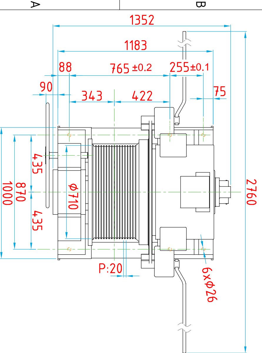
ÜST GÖRÜNÜŞ/TOP VIEW
