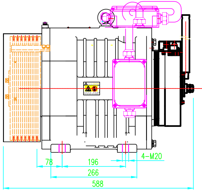
ÖN GÖRÜNÜŞ/FRONT VIEW
