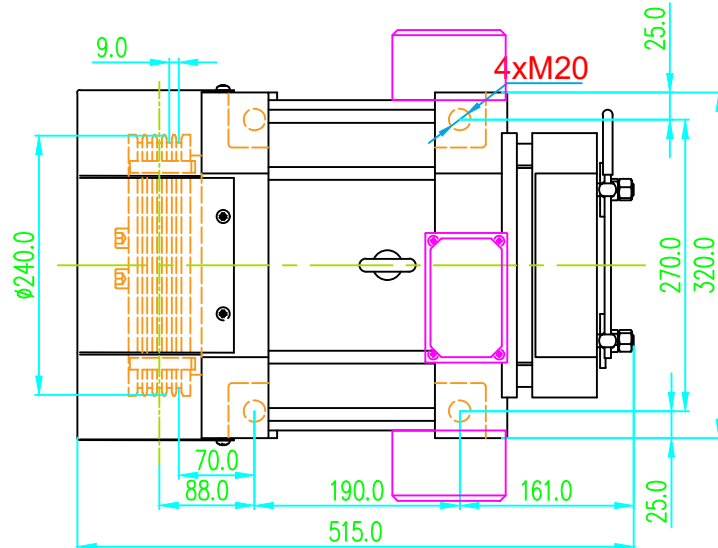
ÜST GÖRÜNÜŞ/TOP VIEW
