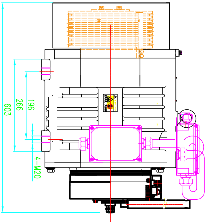
ÖN GÖRÜNÜŞ/FRONT VIEW
